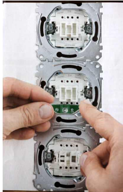
QUICKFLEX® PRÜFKONTAKTE KOMFORTABEL PRÜFEN VON VORNE
